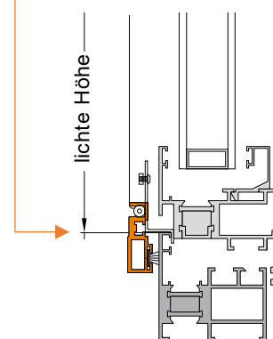
Unterkante des Blendrahmens bei Alufenster flächenbündig
