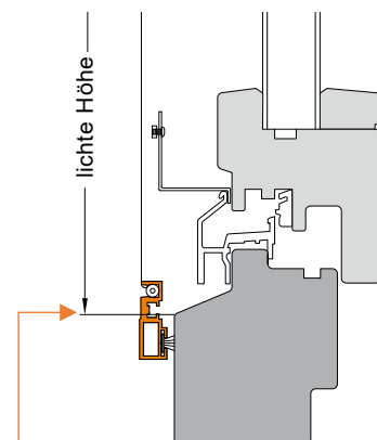
Unterkante des Blendrahmens bei Holzfenster flächenversetzt
