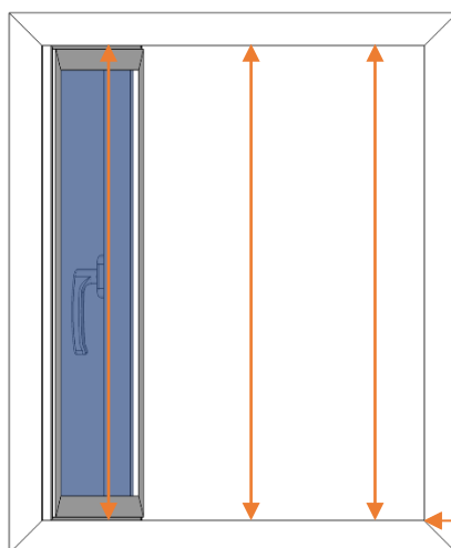
Unterkante des Blendrahmens bei Holzfenster flächenversetzt
