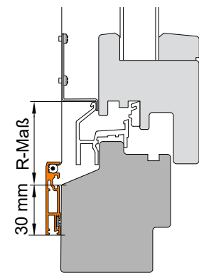
R-Maß bei Holzfenster mit Regenschiene
