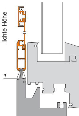
Oberkante des Blendrahmens bei Kunststofftür flächenversetzt
