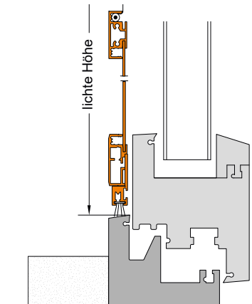
Untere Auflage Laibung bei Kunststofftür flächenversetzt
